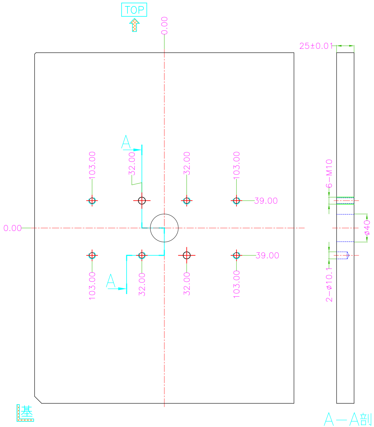
组立板加工图
